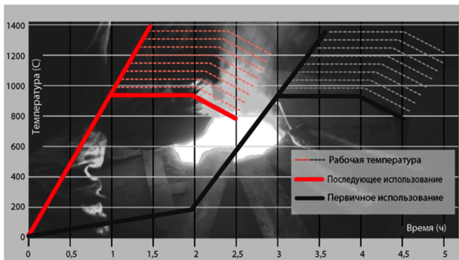
График разогрева карбидокремниевых тиглей марки STARRBIDE, OMNIMELT.
