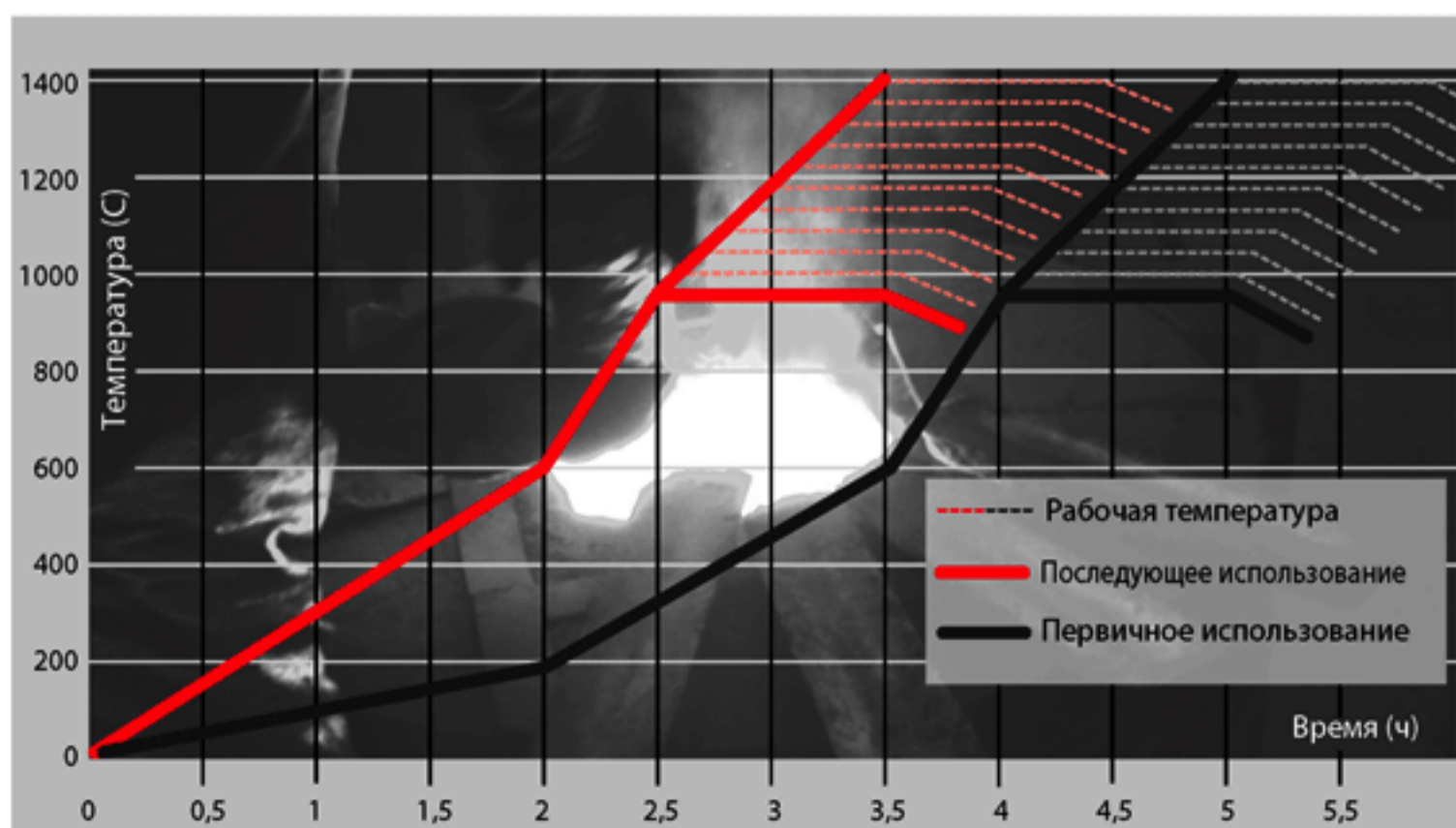
График разогрева графитовых тиглей марки SUPER, ALUSTAR.
